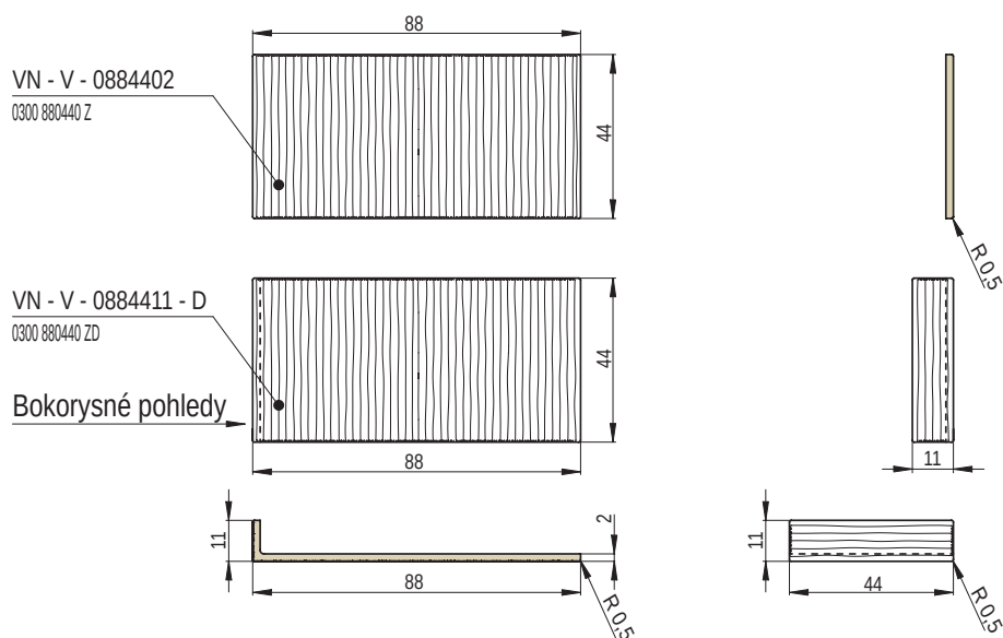
Bokorysné pohledy
