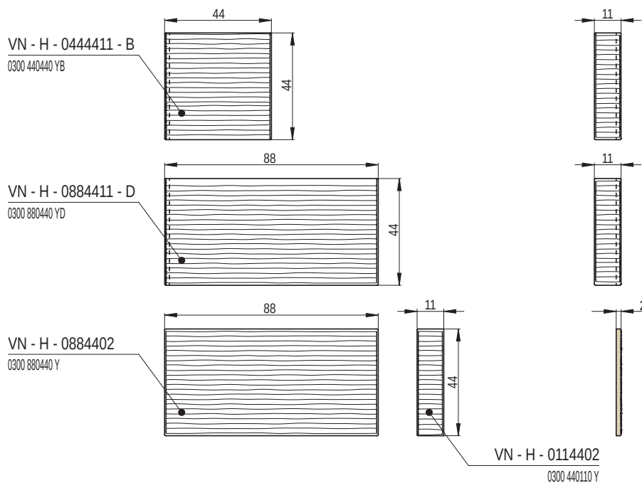
Bokorysné pohledy
